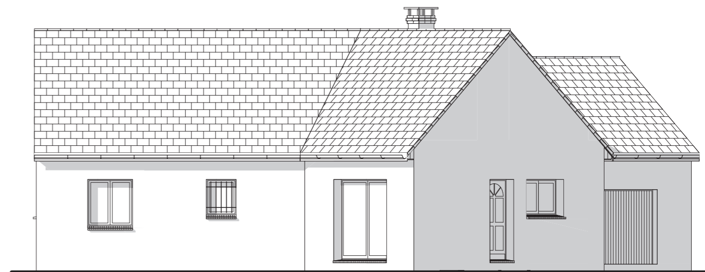
Façade Sud Ouest
