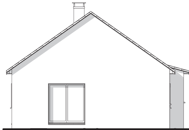
Pignon Nord Est
